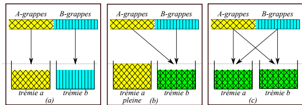
FIGURE 2 – 3 cas possibles pour remplir les trémies. (a) A-grappes et B-grappes sont séparées. (b) quand la trémie a est pleine, les A-grappes et B-grappes sont mixées dans la trémie b . (c) Une fois que R_{min} est atteint, A-grappes et B-grappes sont mélangées dans les deux trémies.
