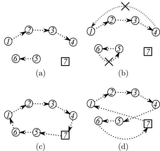
FIGURE 3 – La contrainte de cycle sur les variables successeurs entre les rangs (cercles) et une benne (carré).
